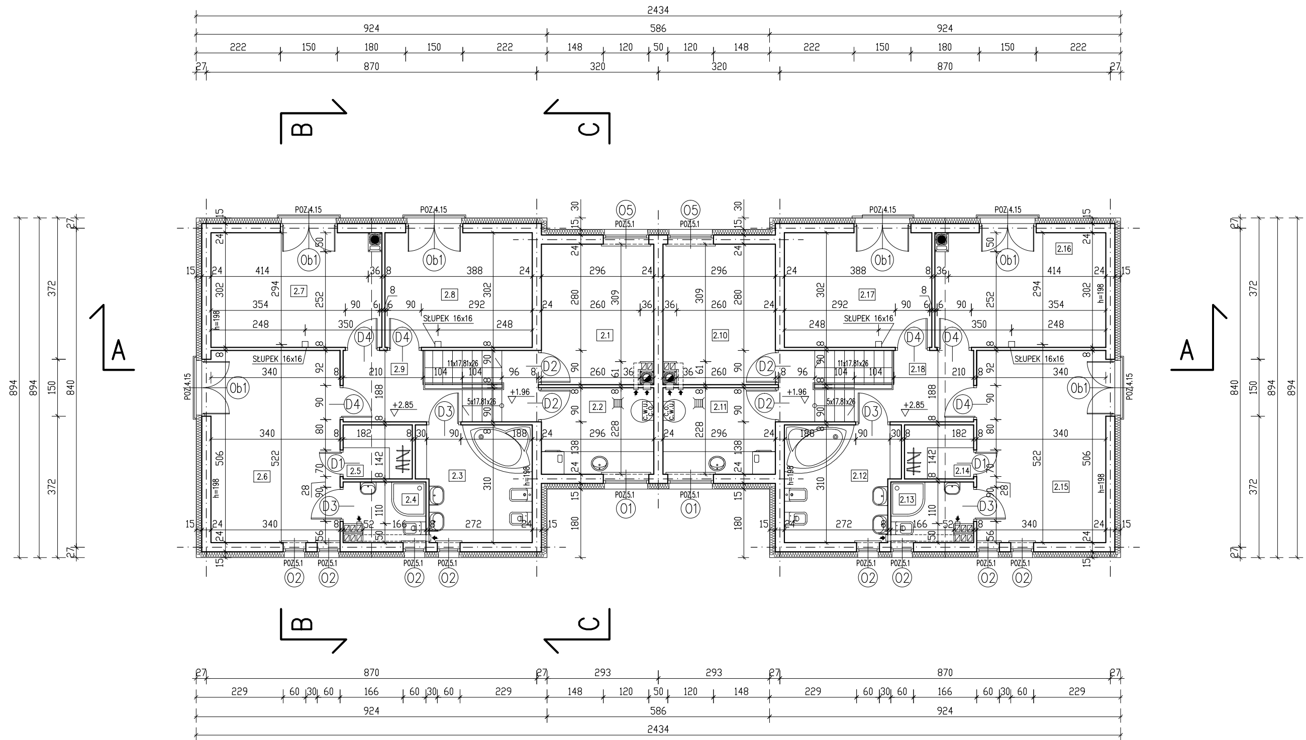
RZUT PODDASZA 1:100
