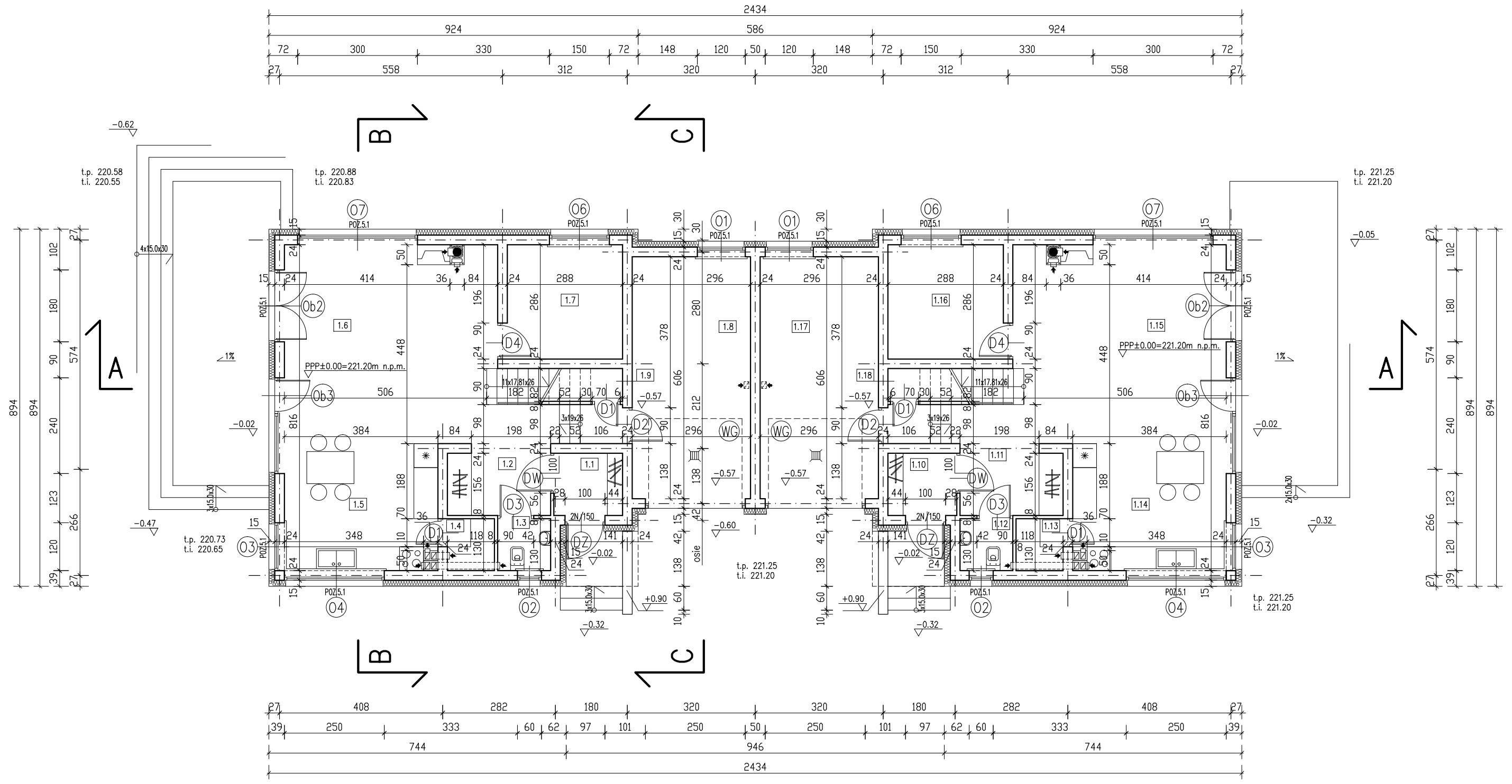
RZUT PARTERU 1:100
